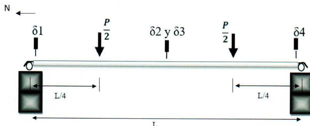
Figura 7.4.1.1. Esquema ensayo a flexión de tablonés.
